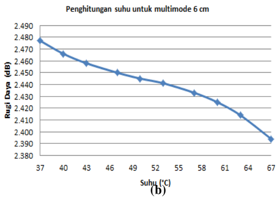
Gambar 3.3. Grafik hubungan rugi daya pada serat optik berstruktur SMS sebagai sensor suhu berdasarkan hasil perhitungan dengan menggunakan metode Interpolasi Lagrange pada panjang serat optik multimode (a) 5,5 cm dan (b) 6 cm.
