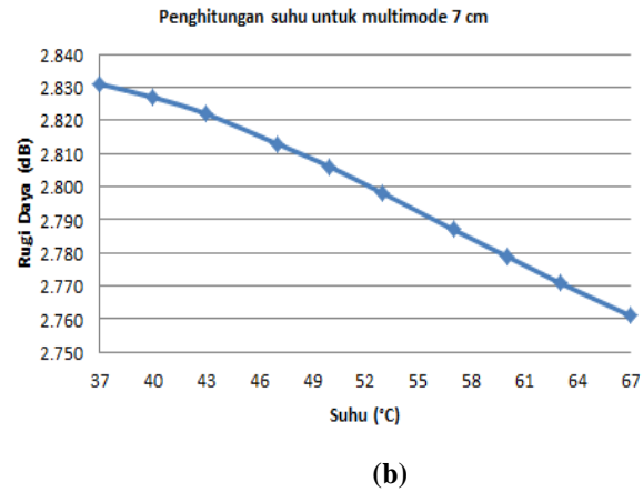
Gambar 3.4. Grafik hubungan rugi daya pada serat optik berstruktur SMS sebagai sensor suhu berdasarkan hasil perhitungan dengan menggunakan metode Interpolasi Lagrange pada panjang serat optik multimode (a) 6,5 cm dan (b) 7 cm.
