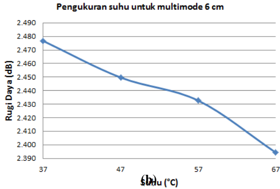
Gambar 3.1. Grafik hubungan rugi daya pada serat optik berstruktur SMS sebagai sensor suhu pada panjang gelombang 1310 nm pada panjang serat optik multimode (a) 5,5 cm dan (b) 6 cm.
