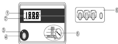
Gambar. 1. Earth Resistance Tester (Diambil dari Manual Instruction : Digital Earth Tester 4105 A)
