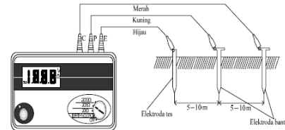
Gambar. 2. Skematik pemasangan elektroda pentanahan dan elektroda bantu untuk proses pengukuran tahanan tanah. (Diambil dari Manual Instruction : Digital Earth Tester 4105 A)
